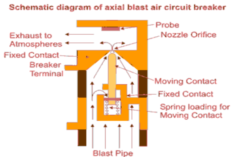
Fig. 1.8 Axial Blast ACB
